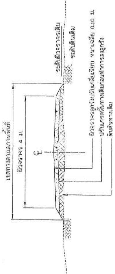
รูปตัดถนนปรับปรุงผิวจราจรลูกรัง มาตราส่วน NOT TO SCALE
